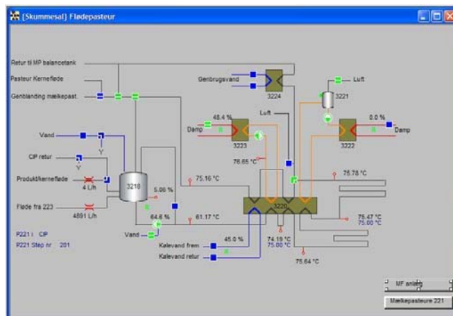
Мнемосхема SCADA системы IGSS
