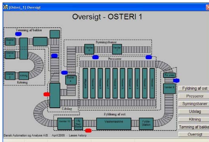
Мнемосхема SCADA системы IGSS
