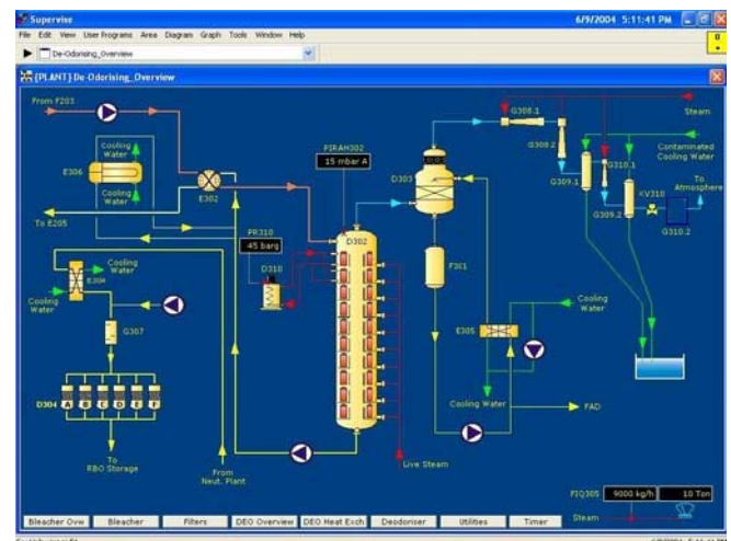
Мнемодиаграмма процесса деодорации
