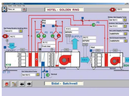
Мнемосхема приточно-вытяжной системы
